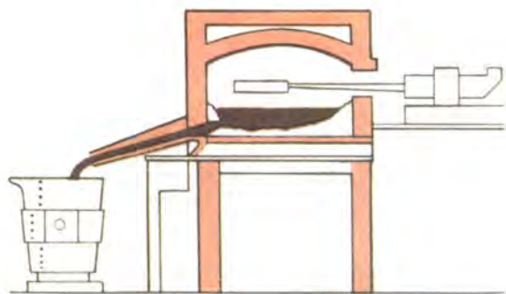
平炉运转示意图
