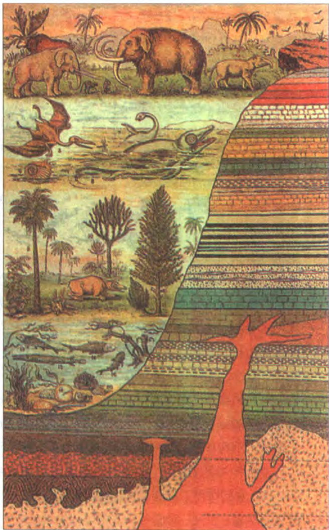
岩石的结构和生物进化示意图，1880年。
